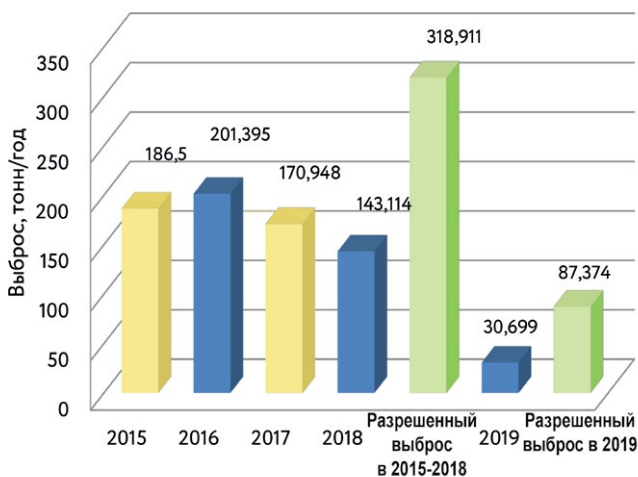
Выброс вредных (загрязняющих) веществ в атмосферный воздух в динамике за 2015-2019 г.г.
