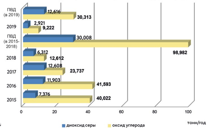
Выбросы диоксида серы и оксида углерода в период 2015-2019 годы в сравнении с нормативами ПДВ, тонн/год
