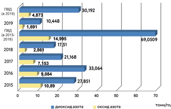
Выбросы диоксида азота и оксида азота в период 2015-2019 годы в сравнении с нормативом, т/г
