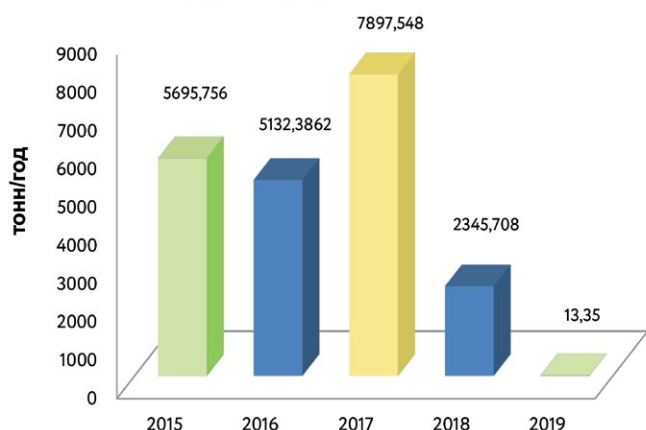
Валовый сброс загрязняющих химических веществ в р. Дон в период с 2015 по 2019 г
