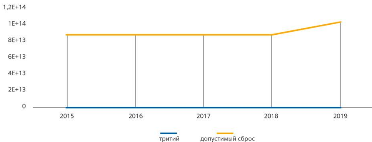
График сброса радионуклида тритий (Бк) с жидкими стоками с 2015 по 2019 годы
