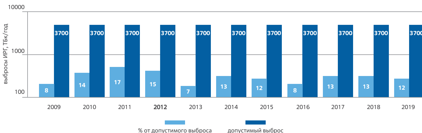
Годовые выбросы ИРГ в период с 2009 по 2019 год
