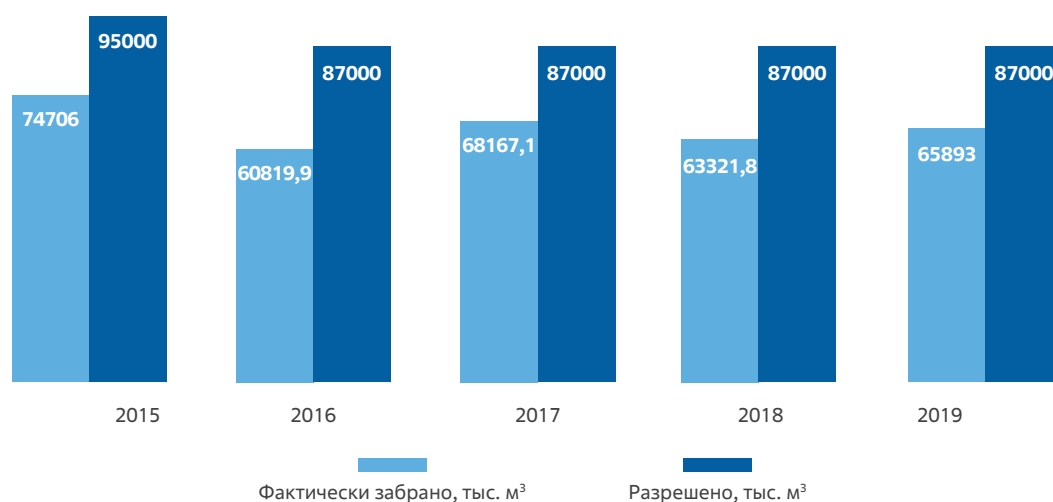
Подпитка водоема-охладителя Курской АЭС
