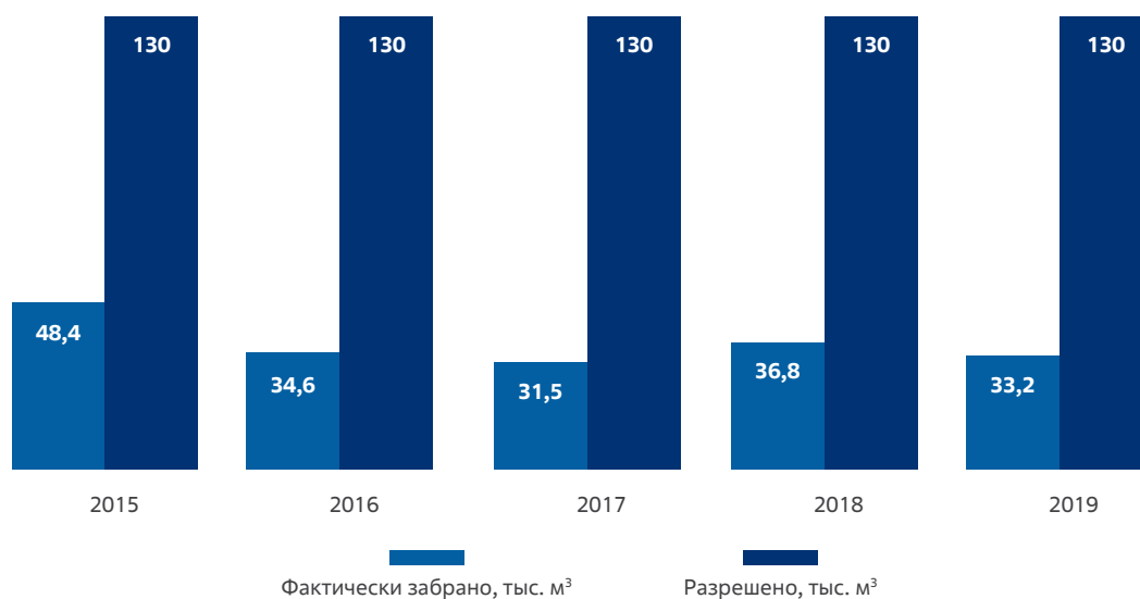
Диаграмма объема забранной воды с/п «Орбита» (подземный горизонт)
