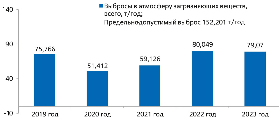
Диаграмма 2. Динамика валовых выбросов вредных химических веществ Смоленской АЭС в атмосферный воздух за последние пять лет
