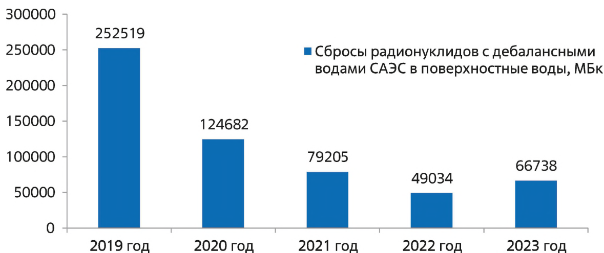
Диаграмма 1. Динамика сбросов радионуклидов с дебалансными водами САЭС в водные объекты за последние пять лет
